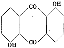
Anthrarufin.
